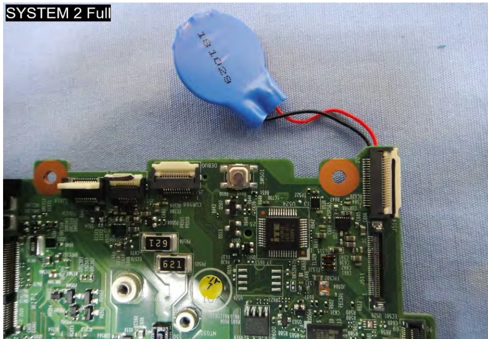
EUT Photo (60)
