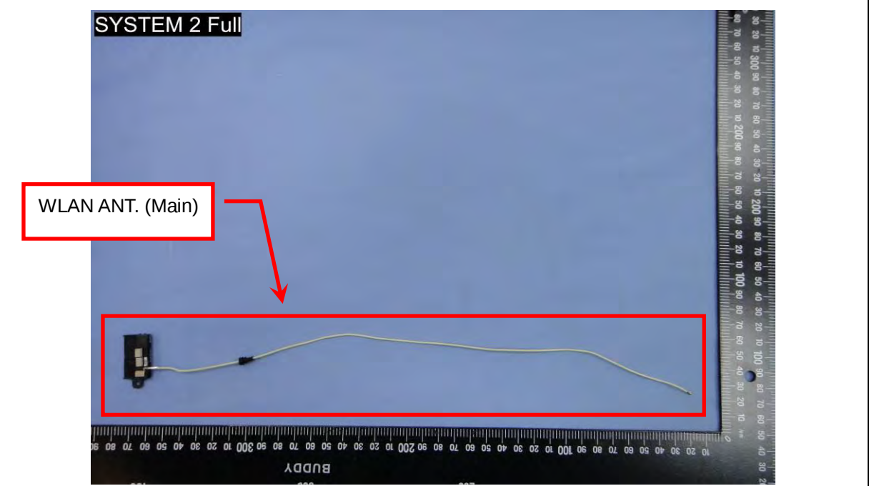
EUT Photo (24)
