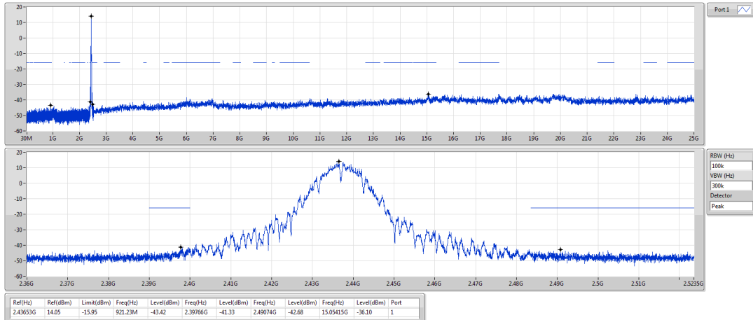
802.11b_Nss1,(1Mbps)_1TX 2437MHz
