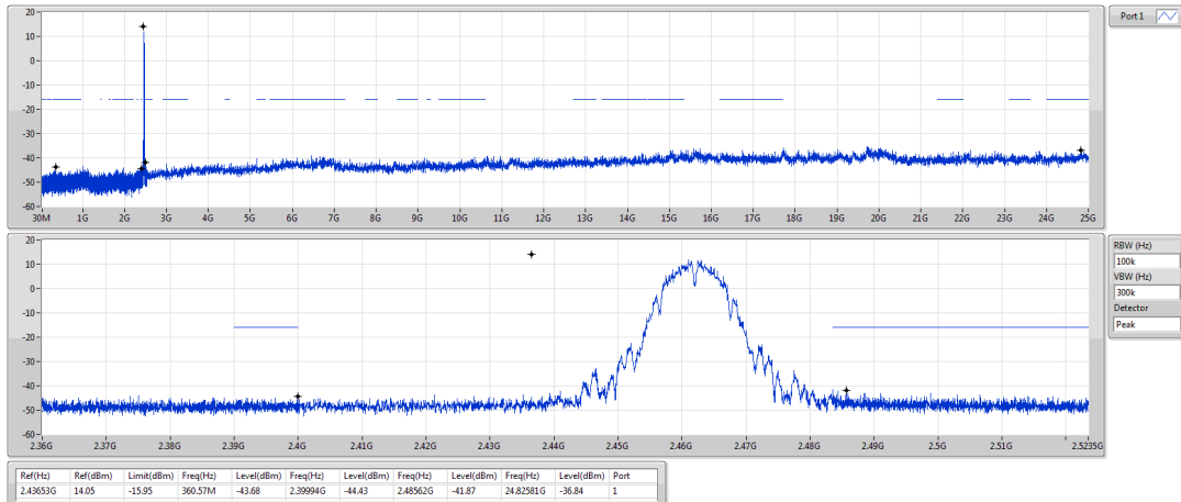
802.11b_Nss1,(1Mbps)_1TX 2462MHz
