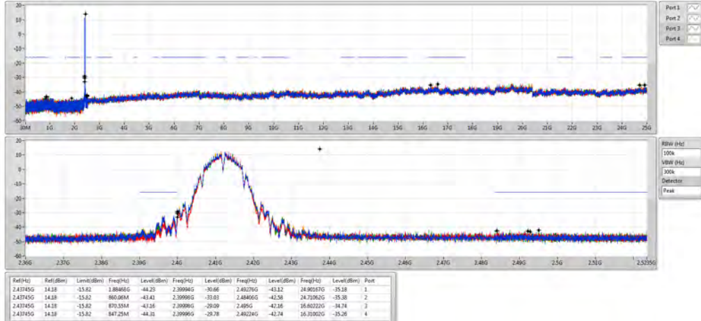
802.11b_Nss1,(1Mbps)_4TX 2412MHz
