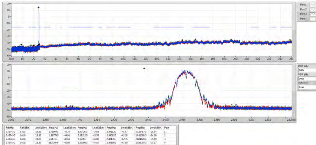
802.11b_Nss1,(1Mbps)_4TX 2462MHz
