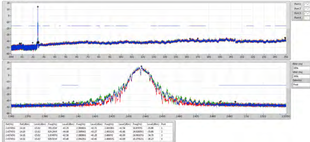
802.11b_Nss1,(1Mbps)_4TX 2437MHz
