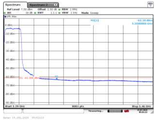
5300MHz with 4*4 CDD AV
