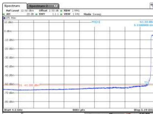
5180MHz with 4*4 Beamforming AV
