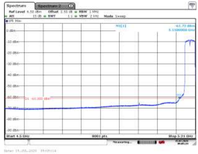
5230MHz with 4*4 CDD AV
