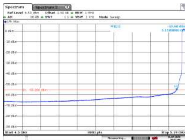
5180MHz with 2*2 Beamforming AV
