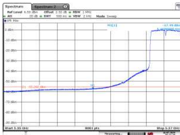
5550MHz with 2*2 CDD AV
