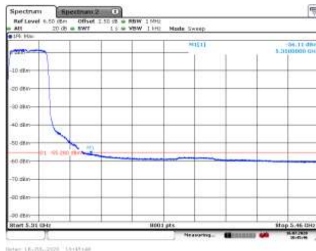
5320MHz with 2*2 Beamforming AV
