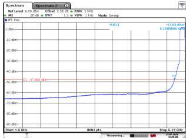
5180MHz AV
