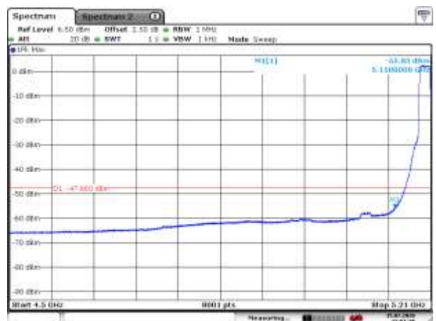
5200MHz AV
