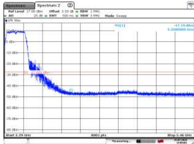
5300MHz PK
