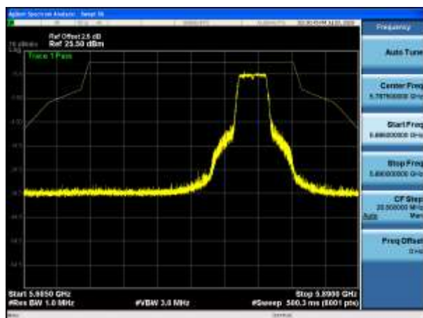
5825MHz PK
