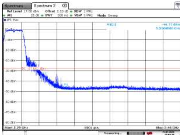
5300MHz PK
