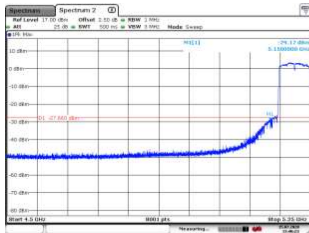
5210MHz PK
