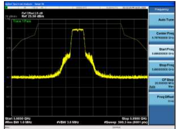
5785MHz PK
