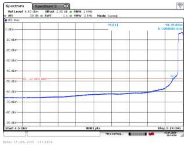
5230MHz AV
