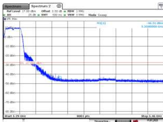
5300MHz PK
