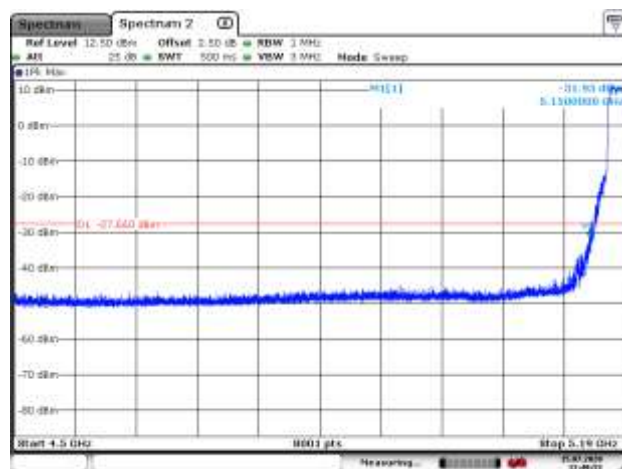
5180MHz PK
