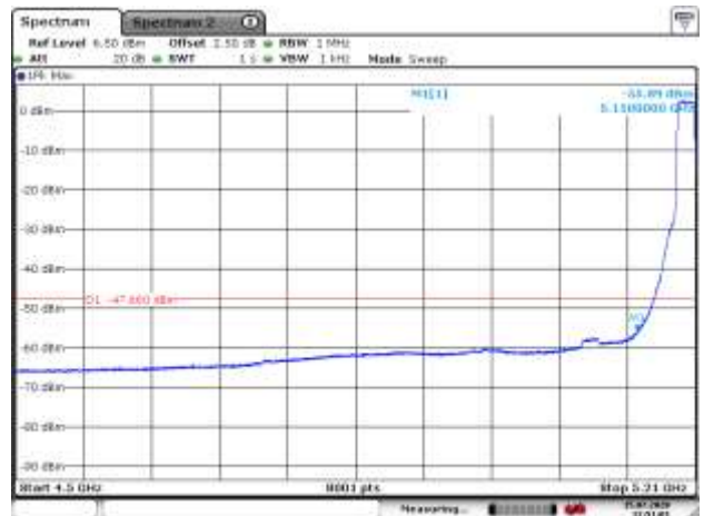
5200MHz AV
