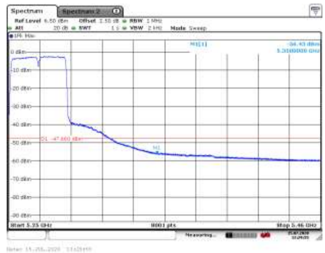
5270MHz AV
