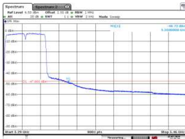
5310MHz AV
