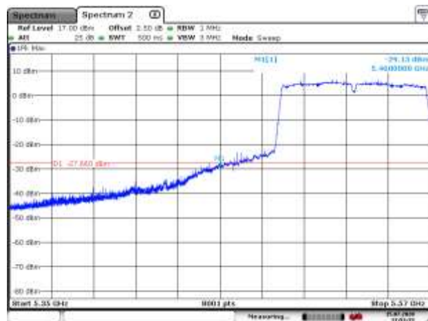
5530MHz PK
