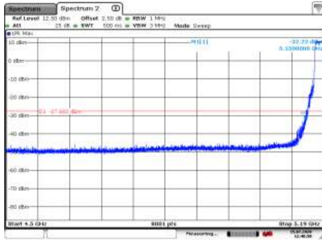
5180MHz PK
