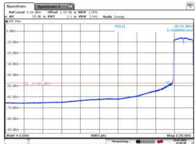
5210MHz AV
