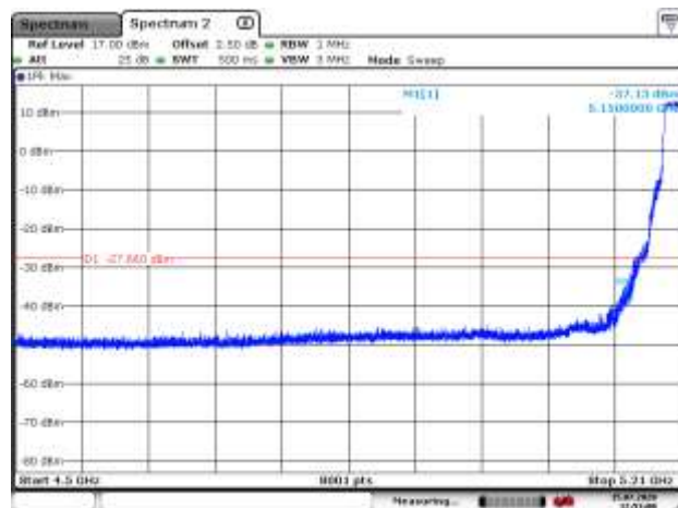
5200MHz PK
