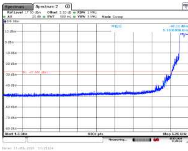
5270MHz PK
