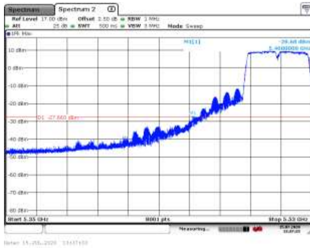
5550MHz PK
