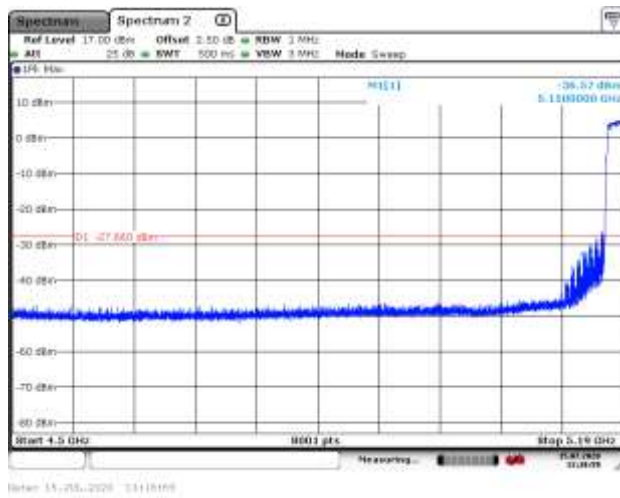
5230MHz PK
