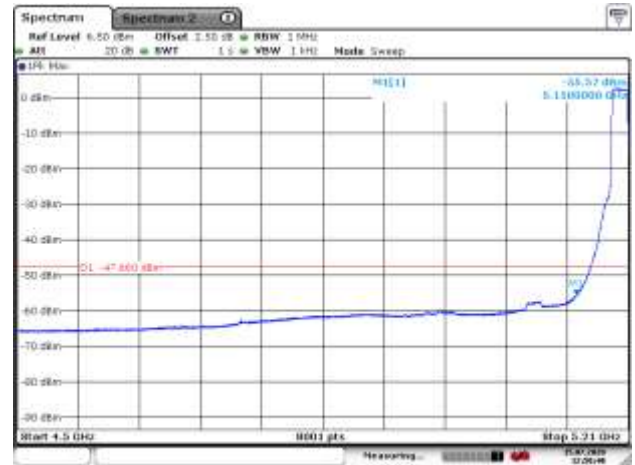
5200MHz AV
