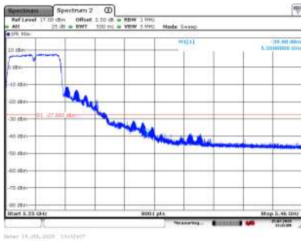
5270MHz PK
