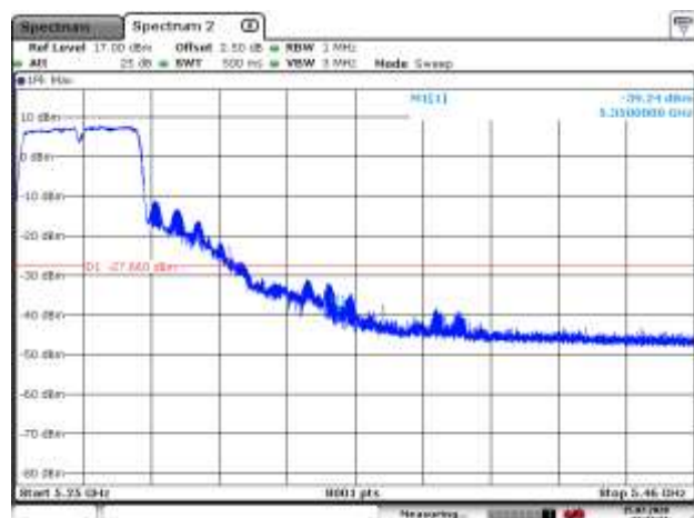
5270MHz PK
