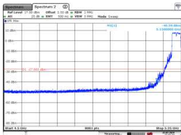
5230MHz PK
