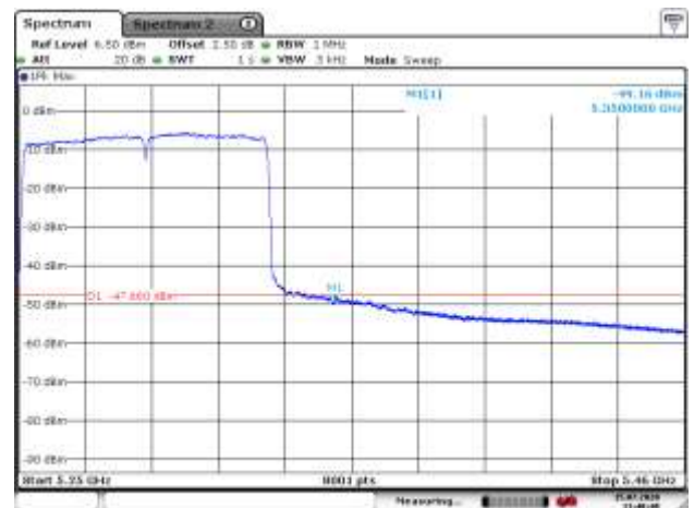
5290MHz AV
