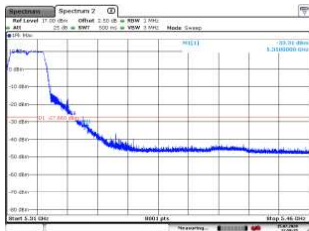
5320MHz PK
