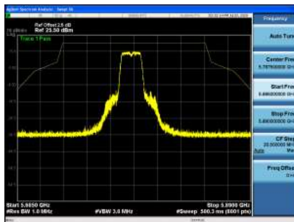
5785MHz PK
