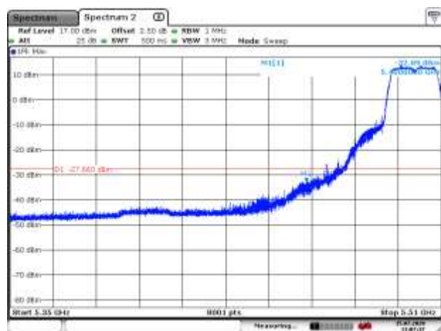
5500MHz PK
