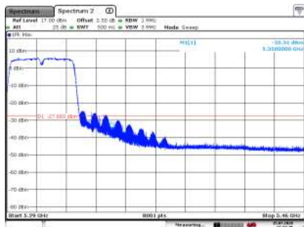
5310MHz PK
