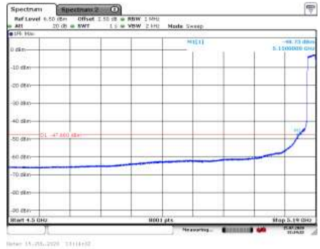
5230MHz AV
