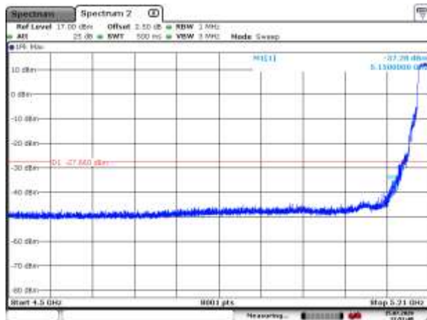
5200MHz PK
