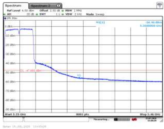
5270MHz AV
