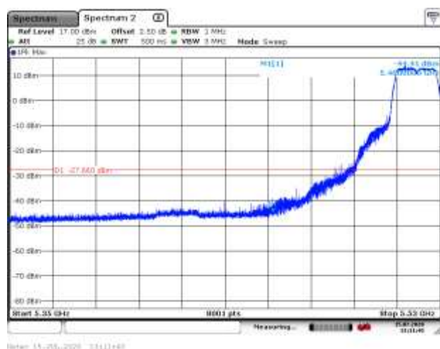
5520MHz PK
