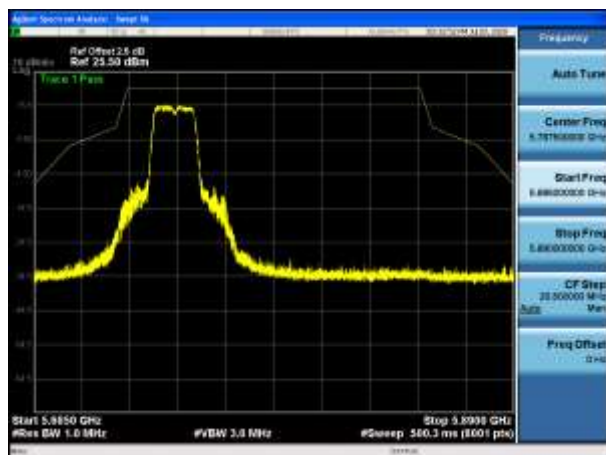
5745MHz PK
