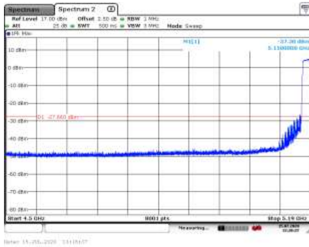
5230MHz PK
