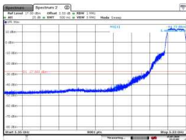
5520MHz PK
