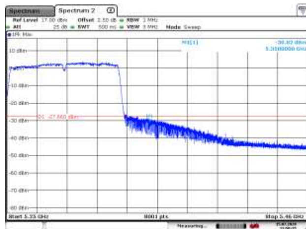
5290MHz PK
