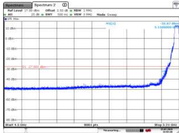
5200MHz PK
