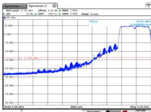
5510MHz PK
