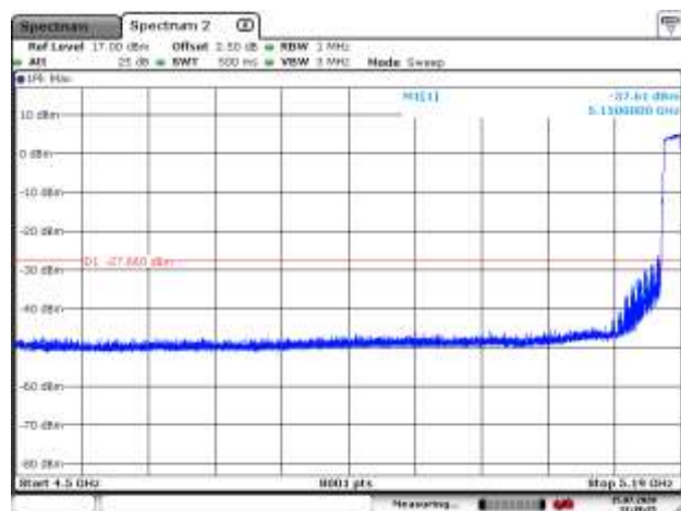
5190MHz PK
