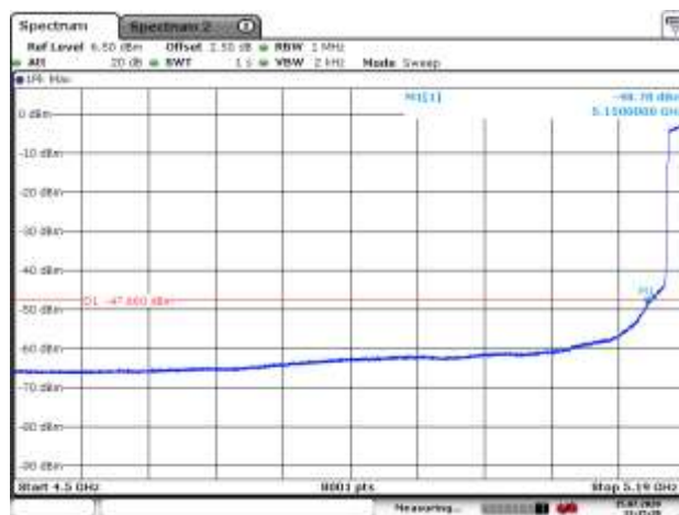
5190MHz AV
