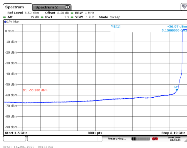
5200MHz with 2*2 CDD AV
