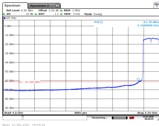
5210MHz with 4*4 Beamforming AV
