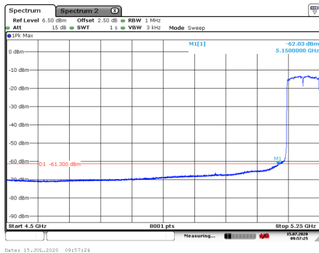
5210MHz with 4*4 CDD AV
