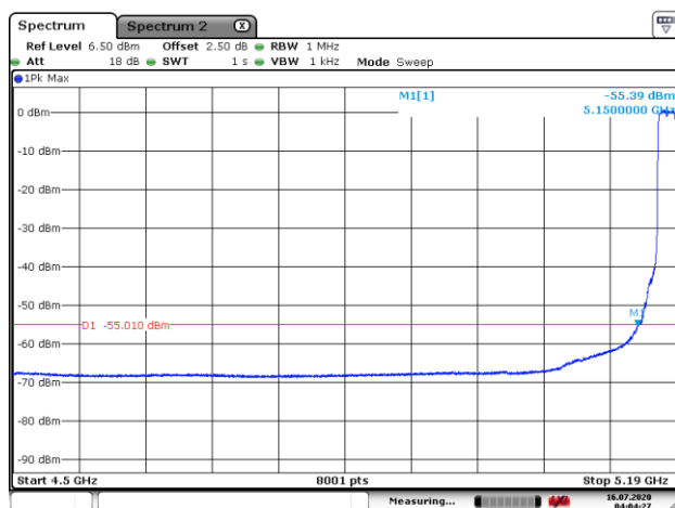
5180MHz with 2*2 CDD AV
