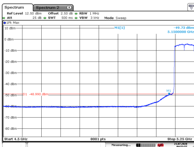
5210MHz with SISO AV
