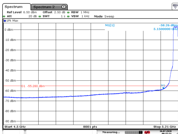
5200MHz with 2*2 CDD AV
