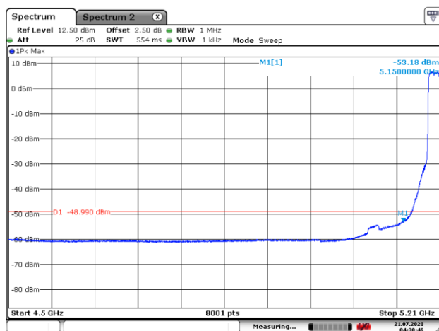
5200MHz with SISO AV
