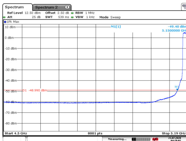
5180MHz with SISO AV
