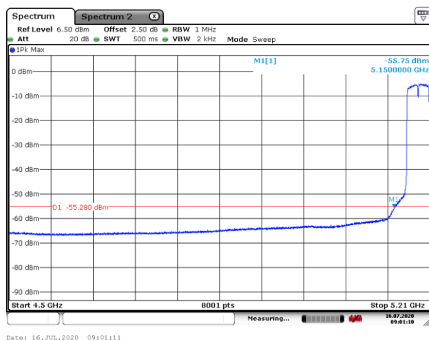
5230MHz with 2*2 CDD AV
