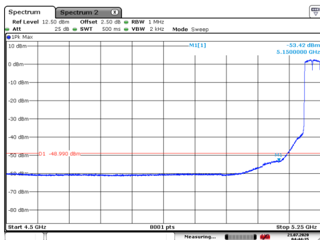
5230MHz with SISO AV
