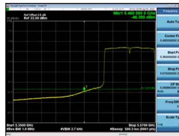
5530MHz AV
