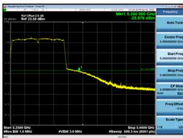
5290MHz PK
