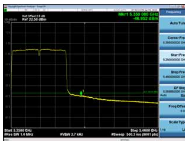
5290MHz AV
