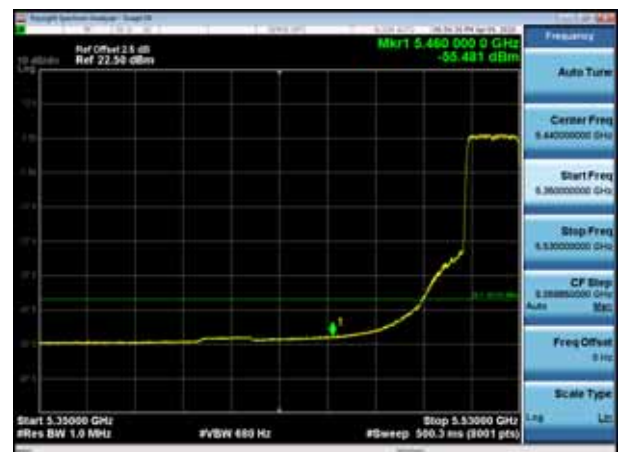
5520MHz AV
