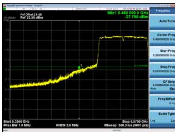
5530MHz PK
