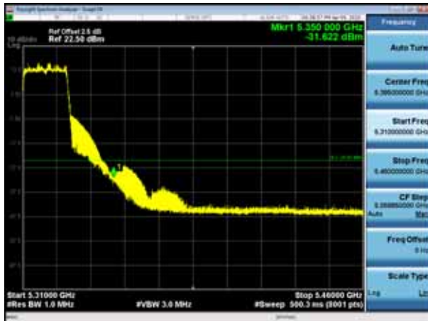
5320MHz PK
