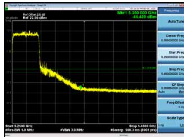
5270MHz PK
