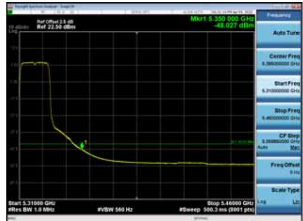
5320MHz AV
