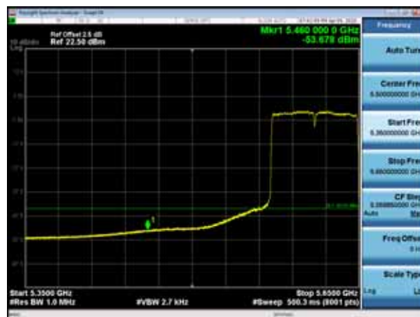
5610MHz AV
