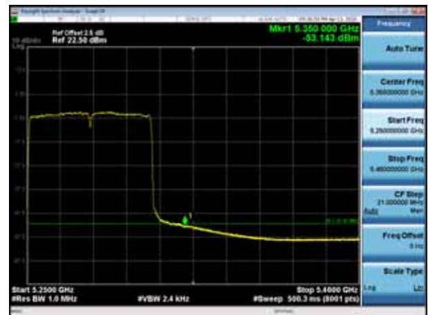
5290MHz with 2*2 Beamforming AV
