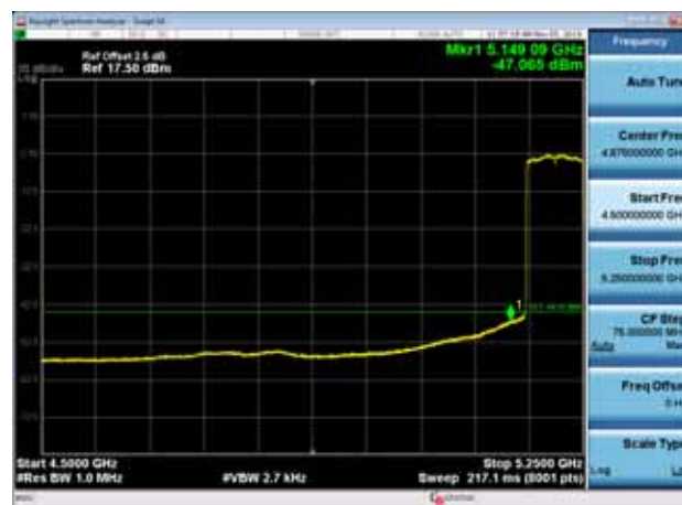
5210MHz AV
