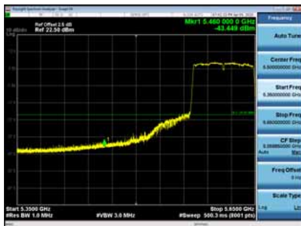
5610MHz PK
