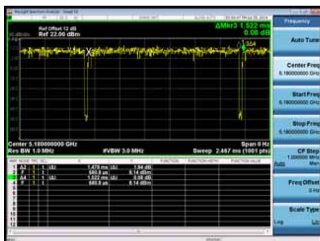
802.11ax(20MHz)
