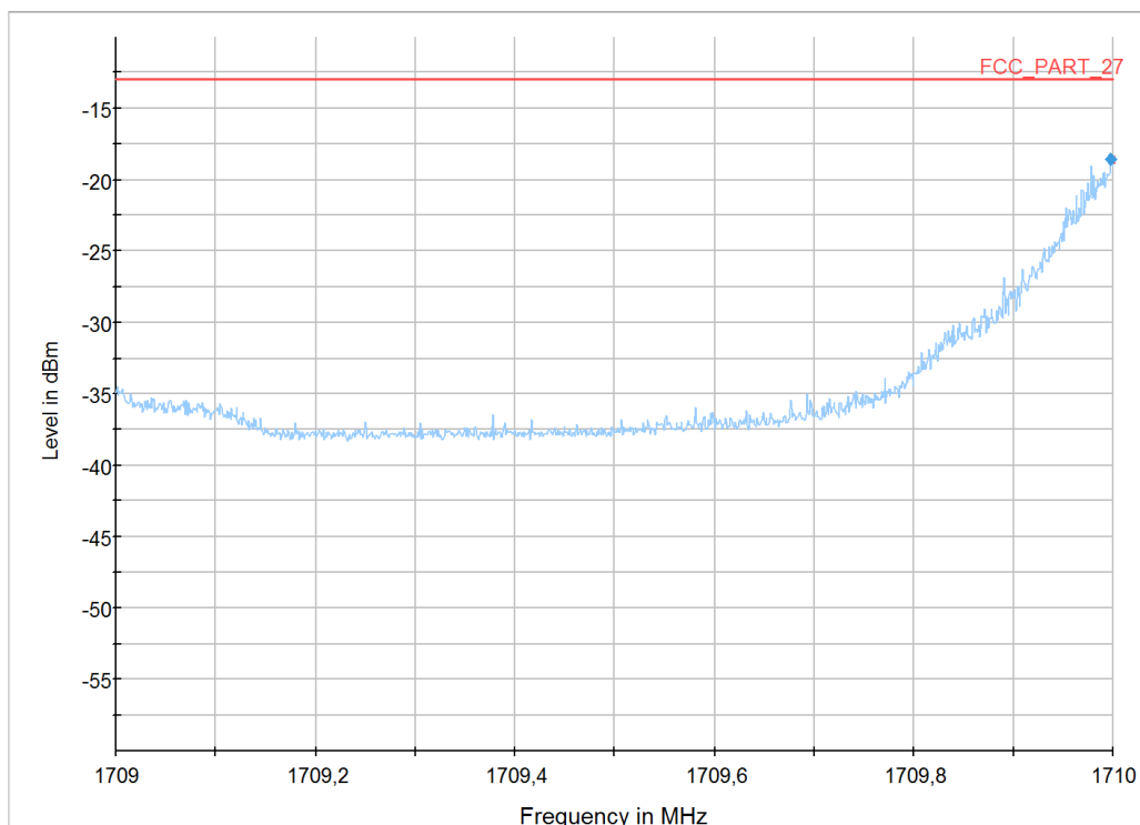
Diagram 17: 9.403a_LTE4_Ch19965_RB1low_BW3MHz_QPSK
