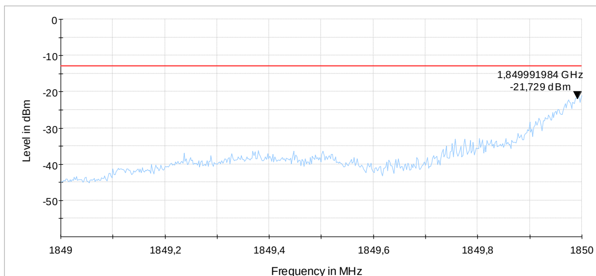
Diagram 9.20a_Ch18607BW_1.4MHz_1RBlow_QPSK
