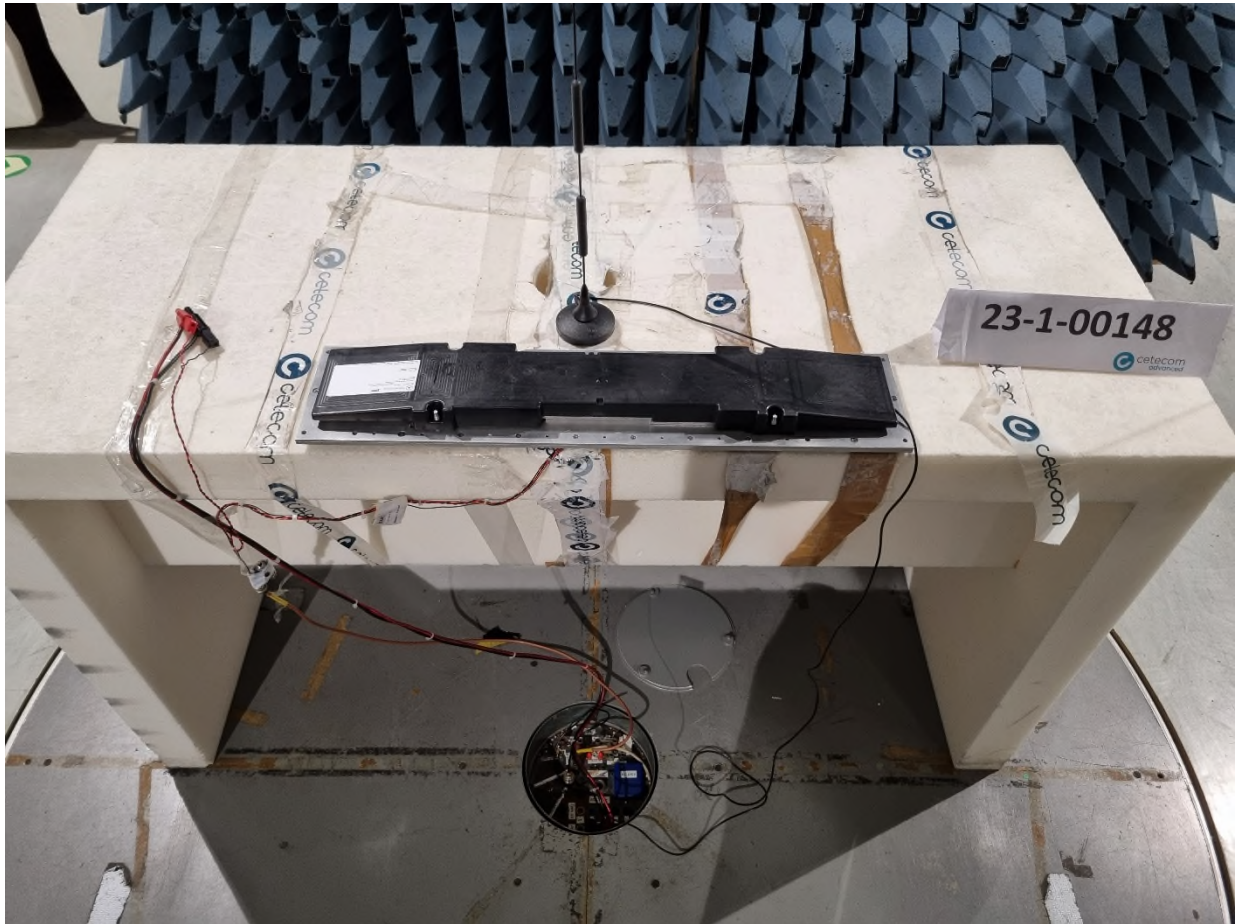
Fig. Mea.: 2 : Radiated RF Parameter Image 2
