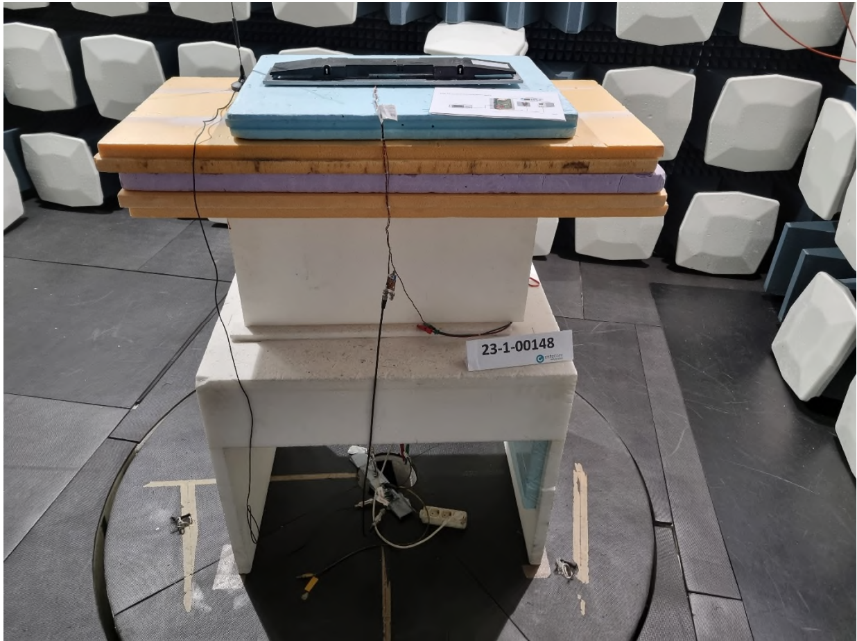
Fig. Mea.: 5 : Radiated RF Parameter Image 5
