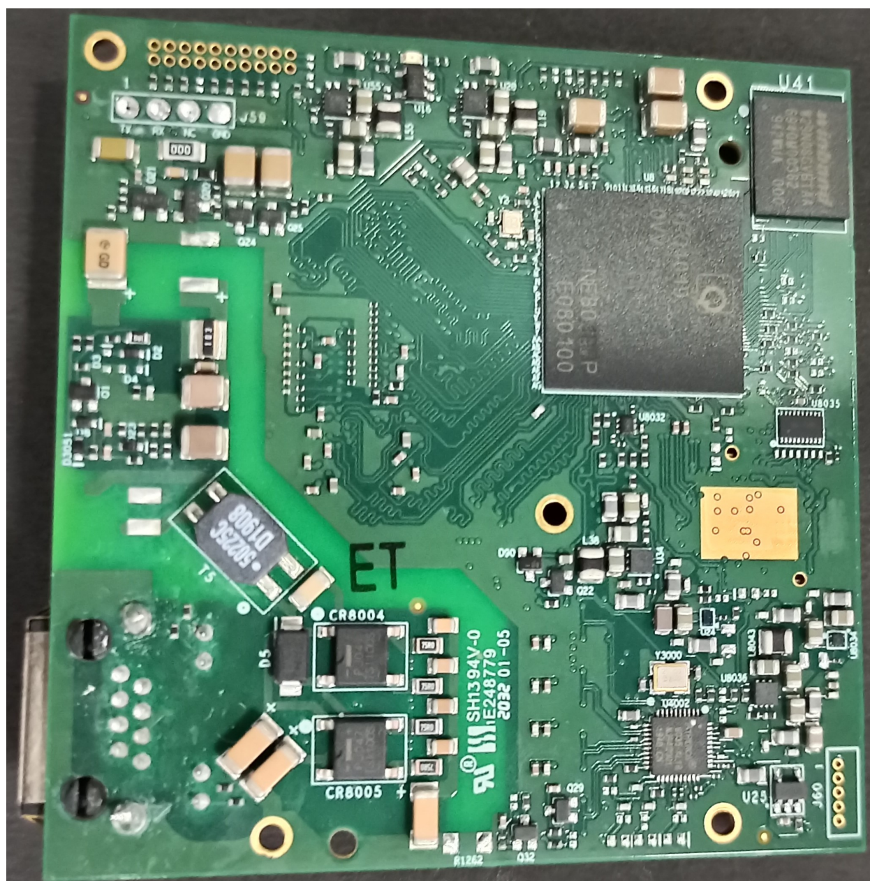
V1000 SSAXA-001001 PCBA Bottom View
