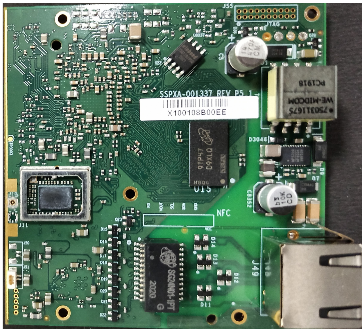
V1000 SSAXA-001001 PCBA Top View
