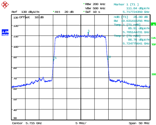
QPSK 5715 MHz
