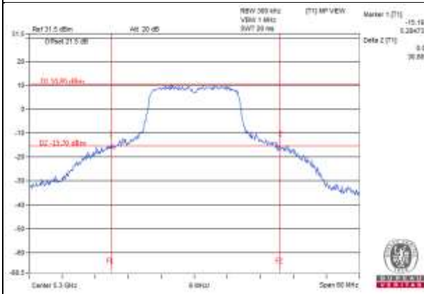
802.11a – CH60
