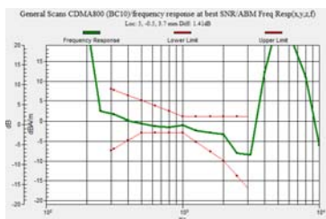
CDMA800 (BC10)
