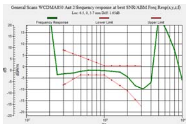
WCDMA850 – Antenna 2
