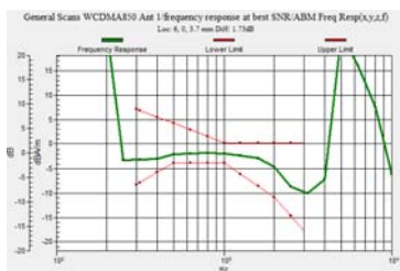
WCDMA850 – Antenna 1
