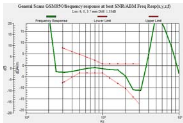
GSM850
