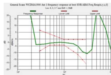
WCDMA1900 – Antenna 1
