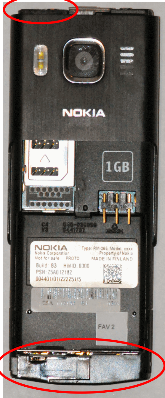
GSM/WCDMA antenna
