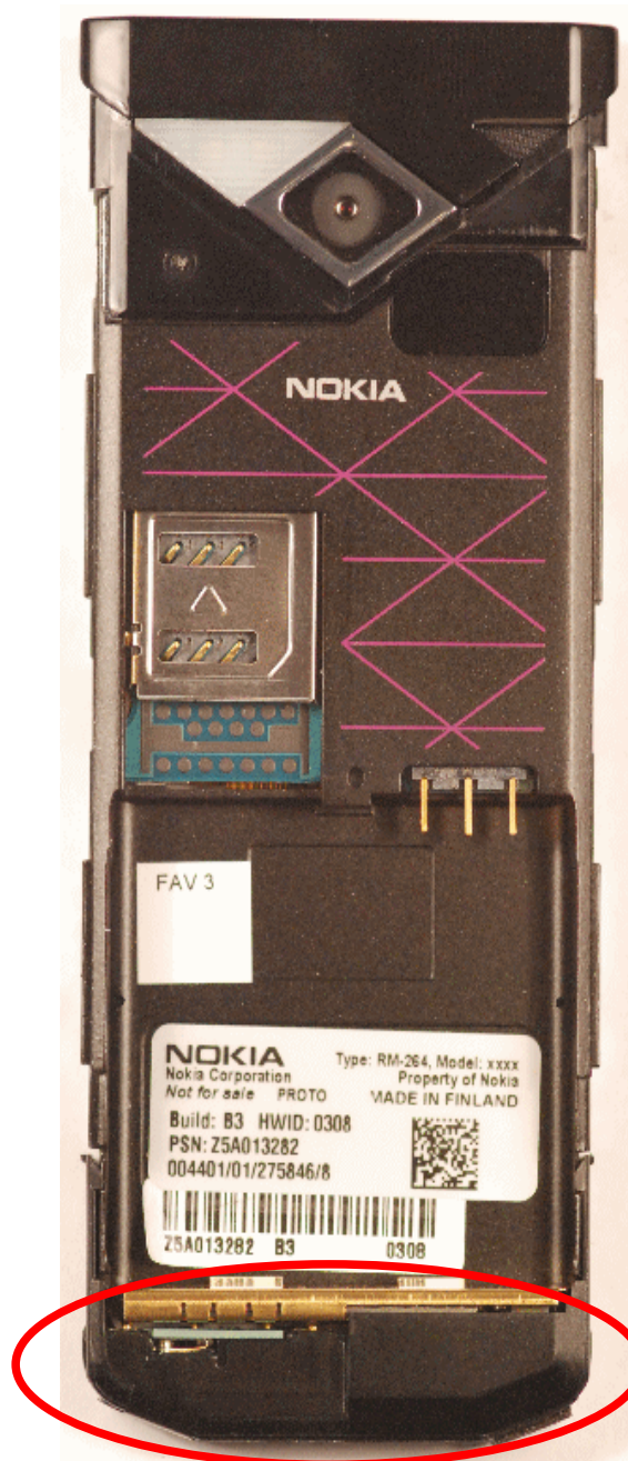
GSM/WCDMA antenna
