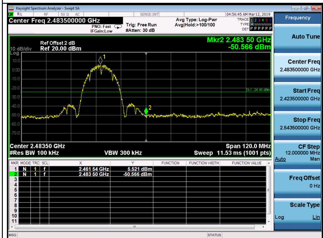
802.11b-2462MHz
