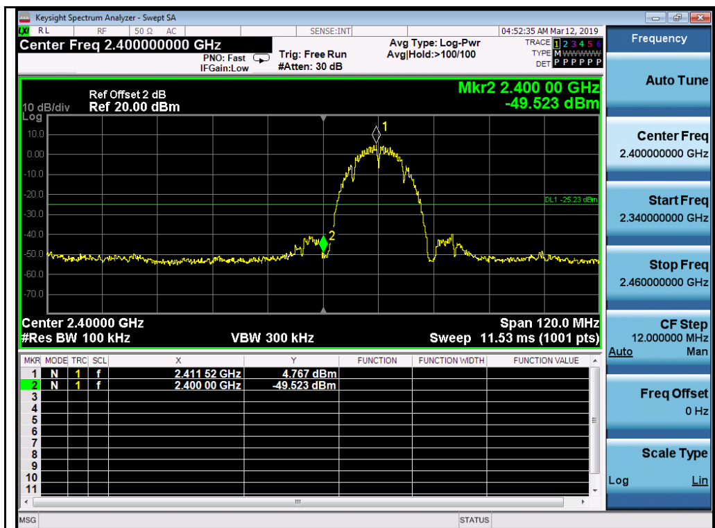
802.11b-2412MHz
