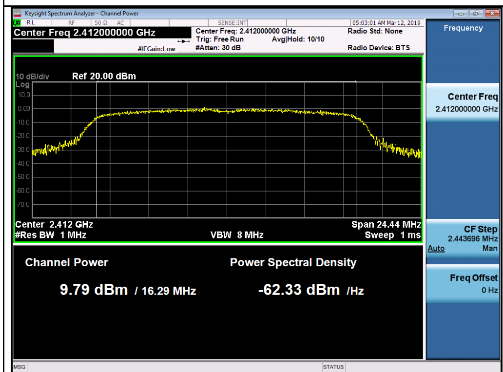
802.11g-2412MHz
