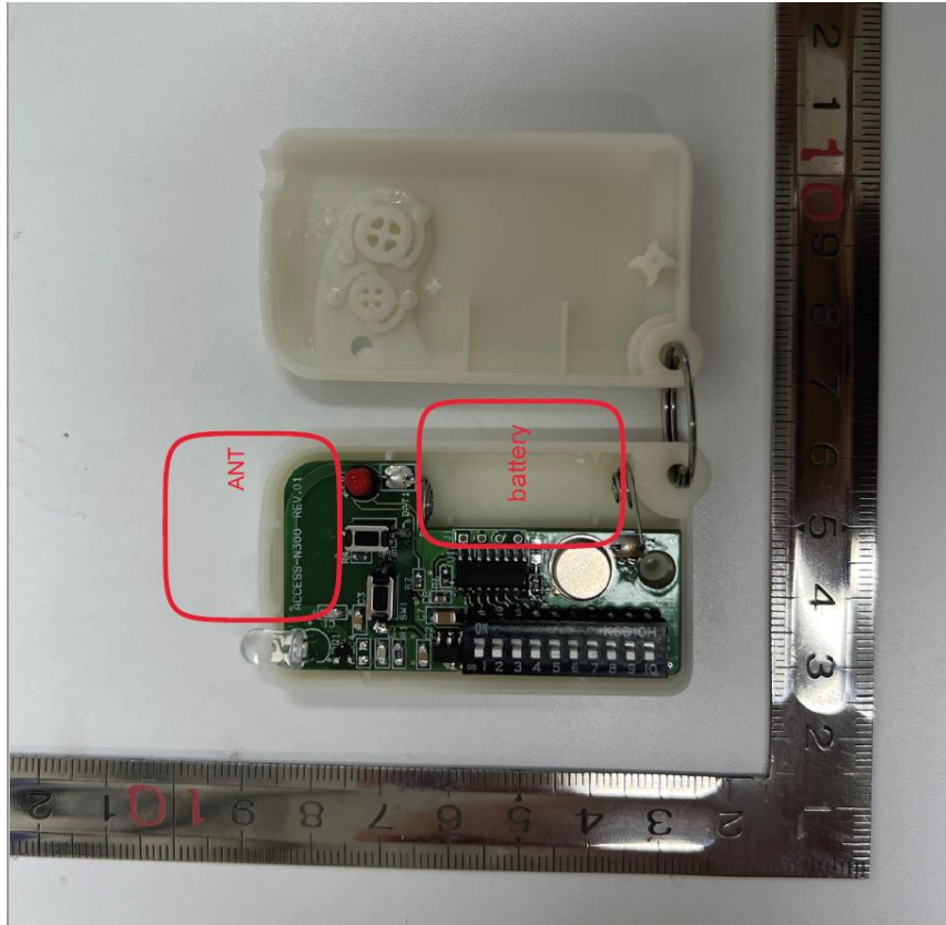
Antenna
