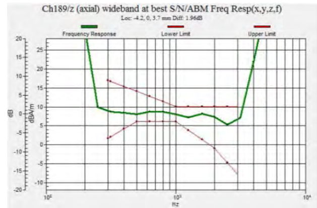
Fig 7.2 GSM850 Ch189
