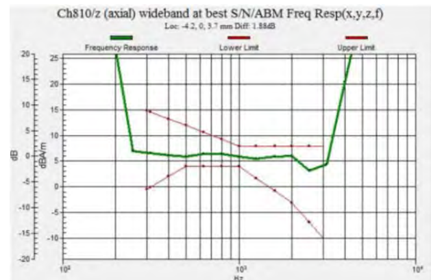
Fig 7.6 GSM1900 Ch810
