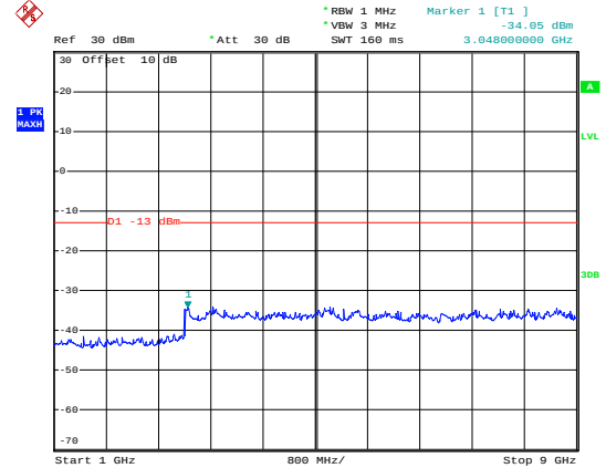
1GHz~9GHz
