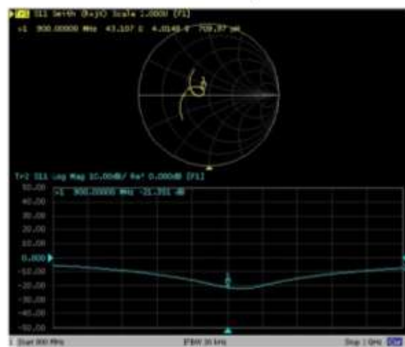
900MHz Body
