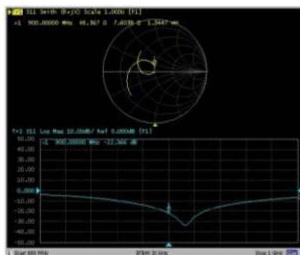
900MHz Head
