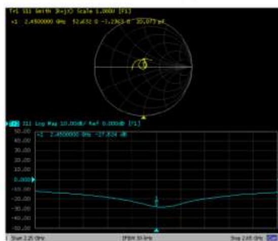
2450MHz Body
