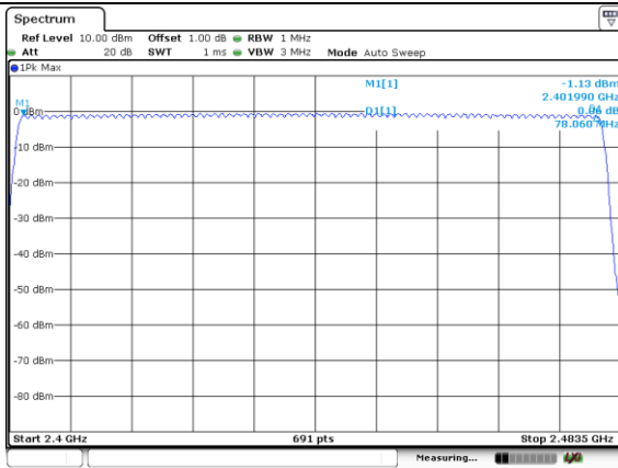
8DPSK
