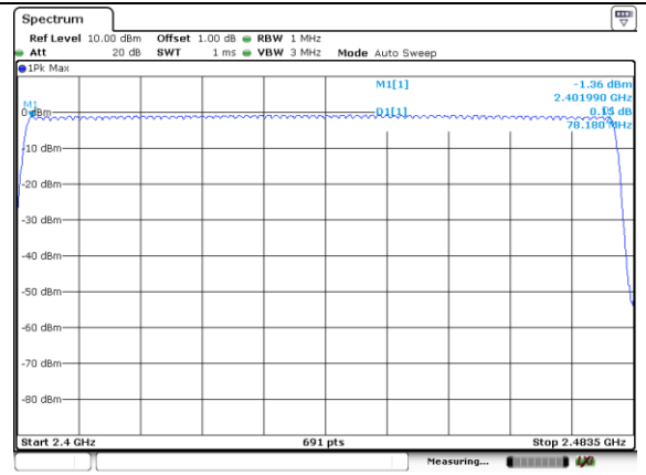
\pi/4 DQPSK
