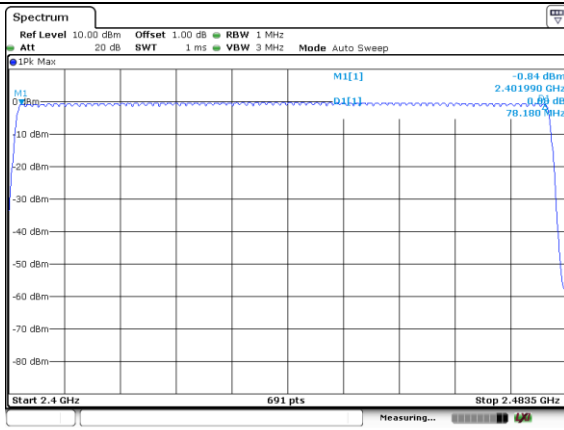
GFSK
