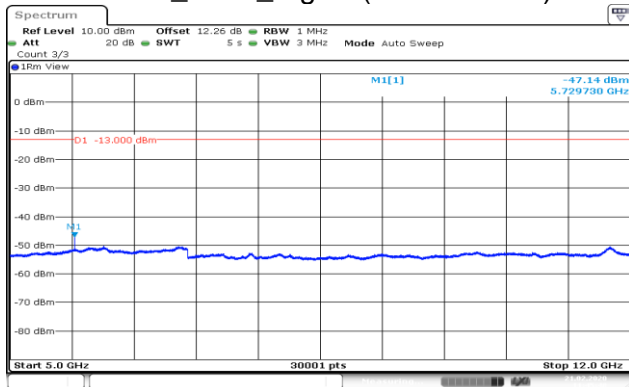
GPRS_1900_Higher(5GHz-12GHz)
