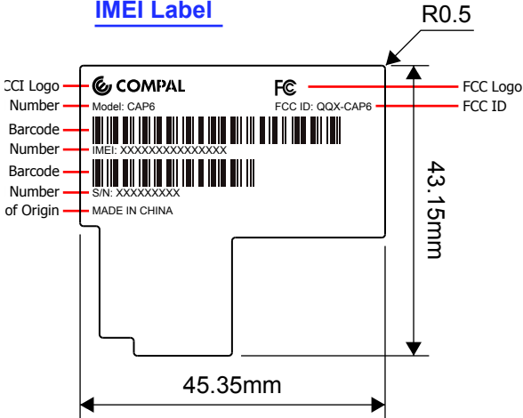
IMEI Label
