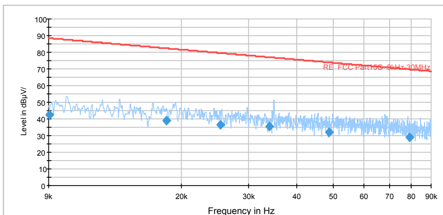
FCC RE 9K-90KHz AV
