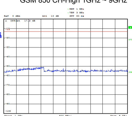
GSM 850 CH-High 1GHz ~ 9GHz
