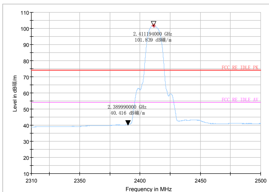
AV detector
