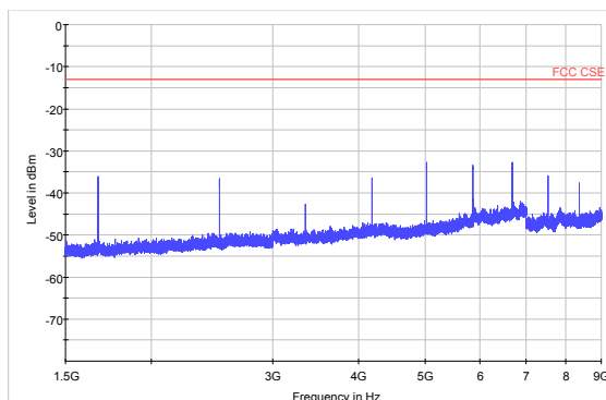
GSM 850 CH-High 1.5GHz ~ 9GHz
