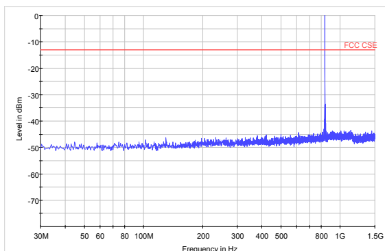
GSM 850 CH-High 30MHz ~ 1.5GHz
