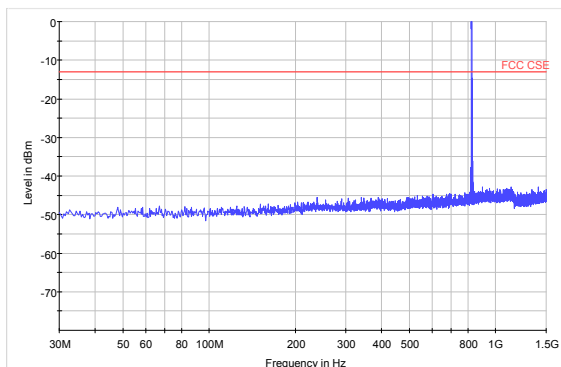
GSM 850 CH-Middle 30MHz ~ 1.5GHz
