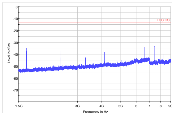
GSM 850 CH-Middle 1.5GHz ~ 9GHz
