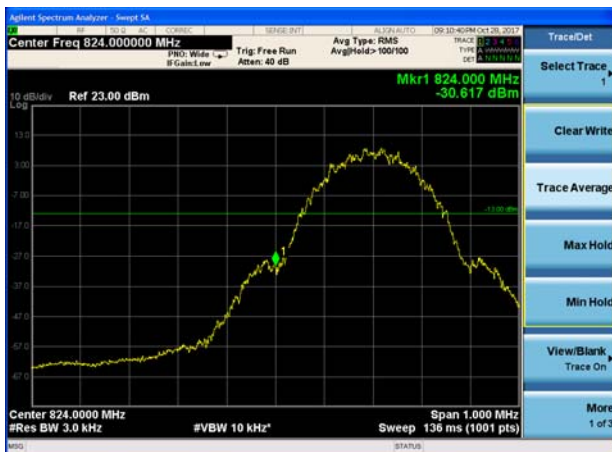
GSM 850 GPRS CH-Low
