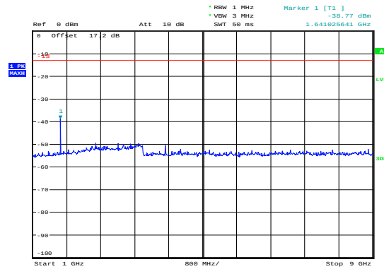
GPRS 850 CH-Low 1GHz ~ 9GHz
