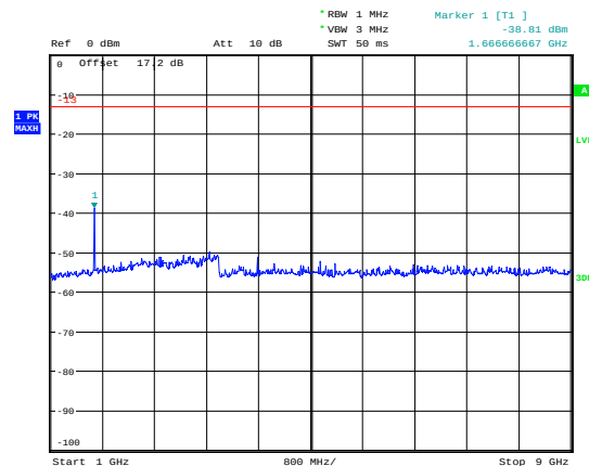
GPRS 850 CH-Middle 1GHz ~ 9GHz
