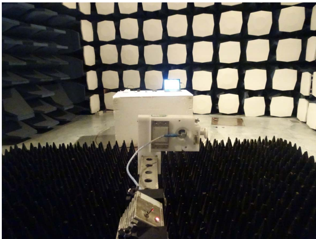
18G-26.5GHz
