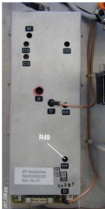
Fig. 4-25 IF Amplifier
