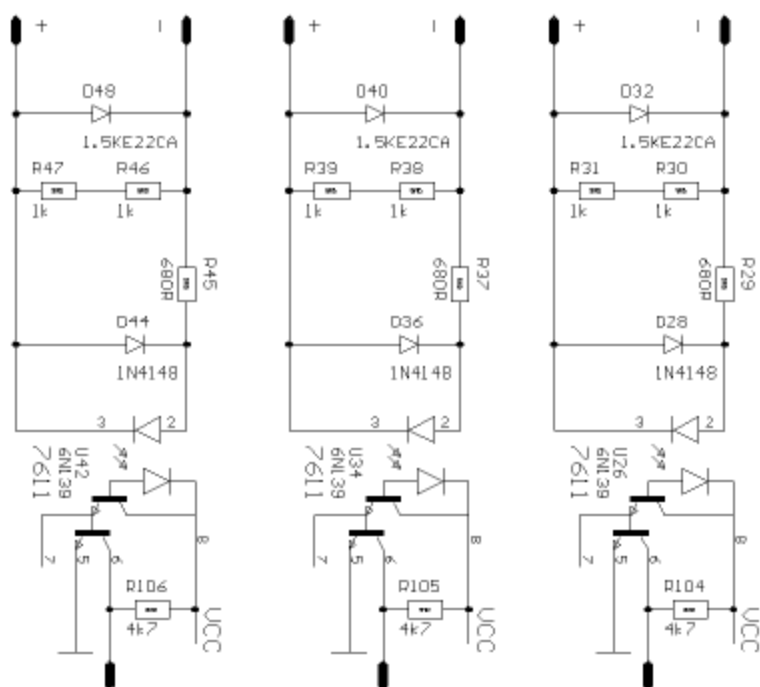
TTL-Seite/serielle Schnittstellen
