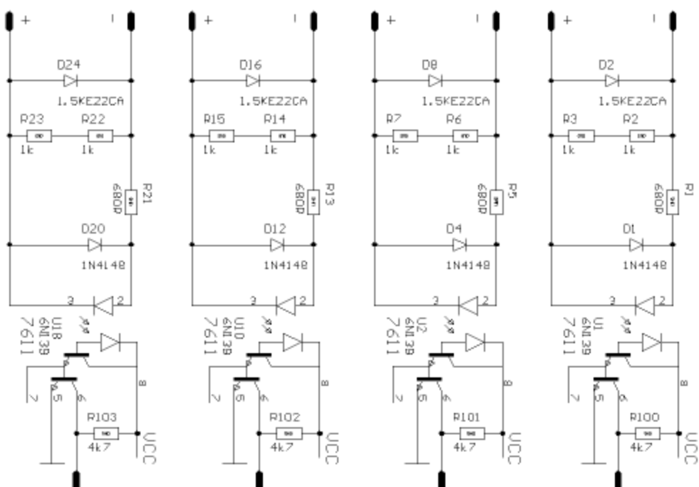
TTL-Seite/serielle Schnittstellen
