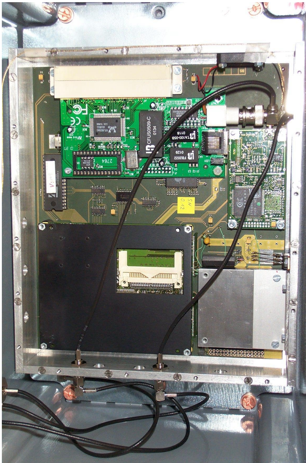
20273eut20.jpg DEBEG 3400, Microcontoller part
