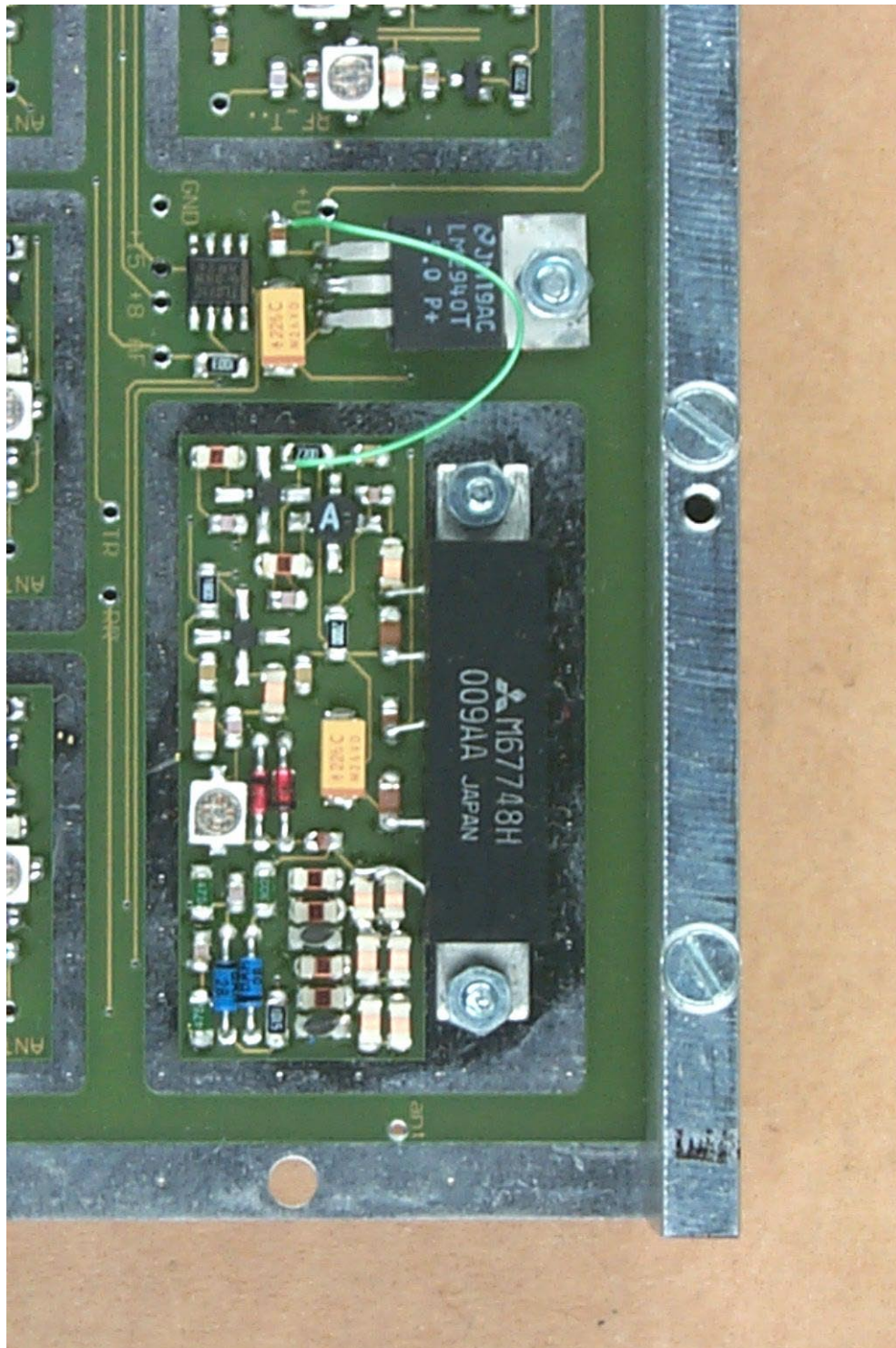
20273eut12.jpg DEBEG 3400, PCB, RF-power-amplifier
