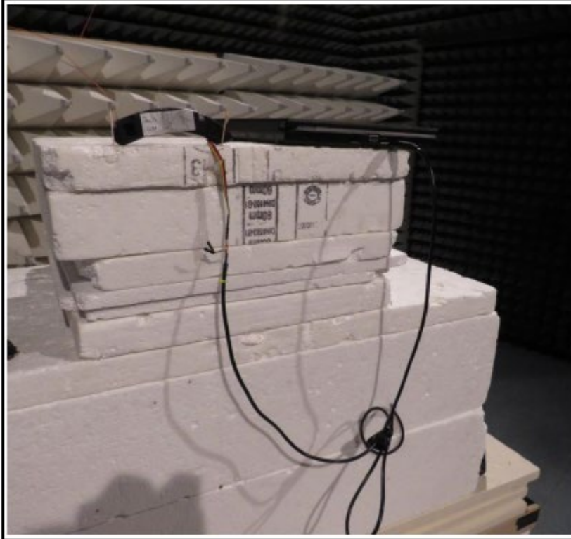
EUT Test Setup (EUT horizontal 1)
