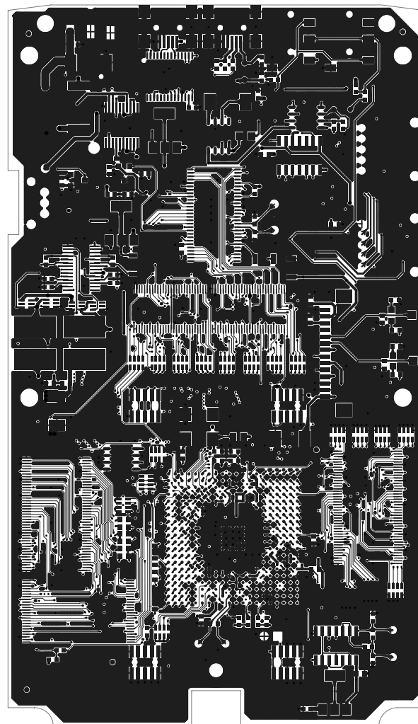
TOP LAYER
