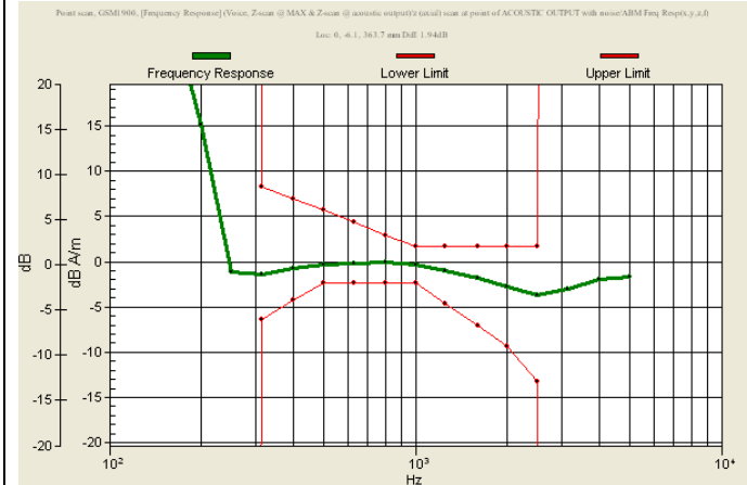
GSM1900
