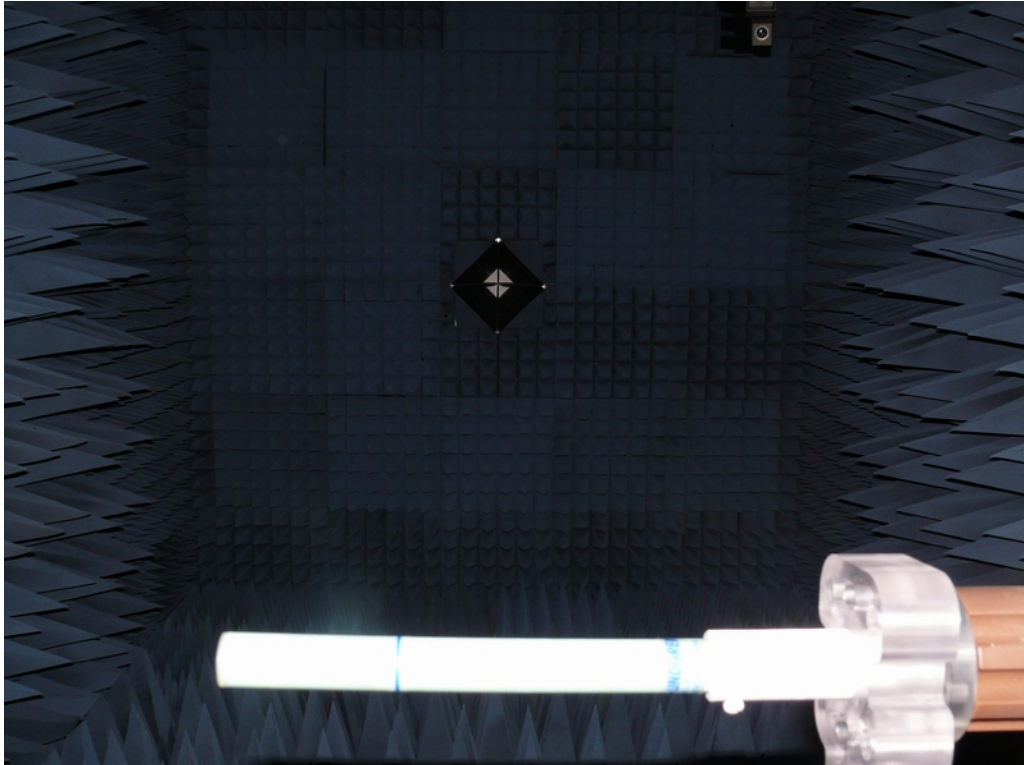
E.R.P. Test Step 1 test setup
