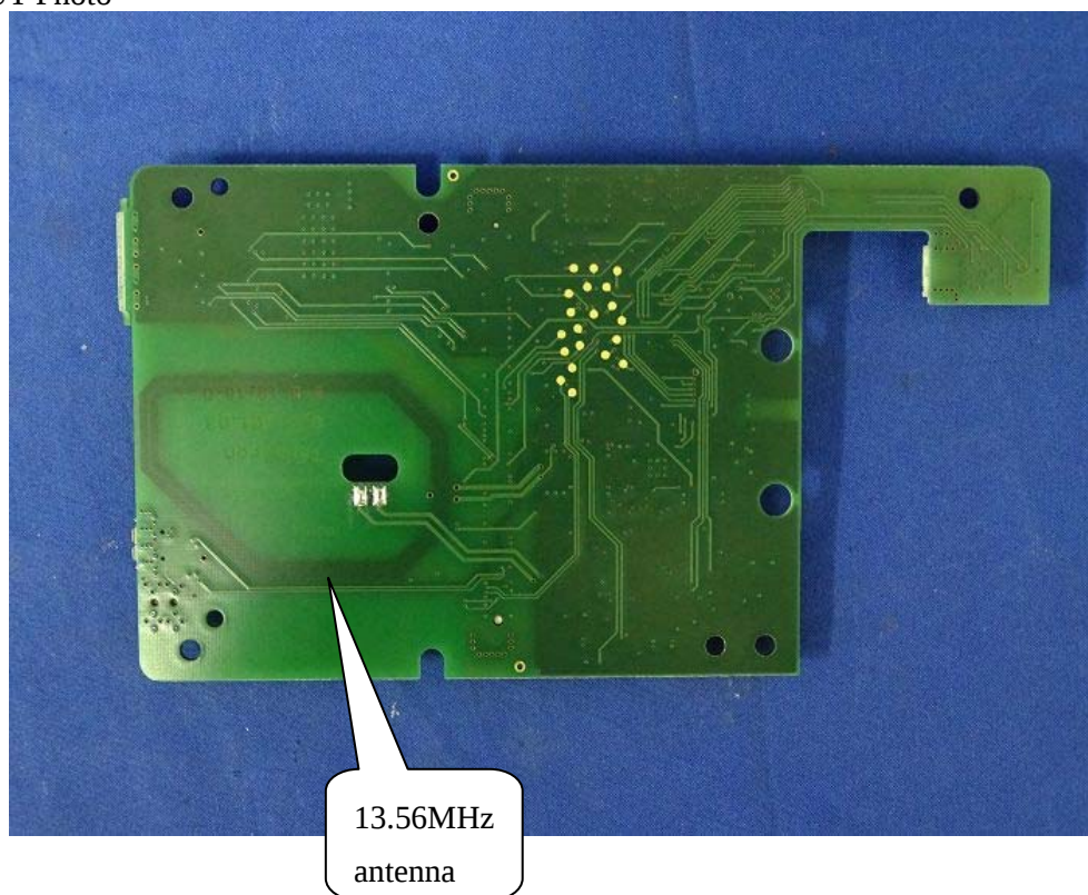
(20) EUT Photo
