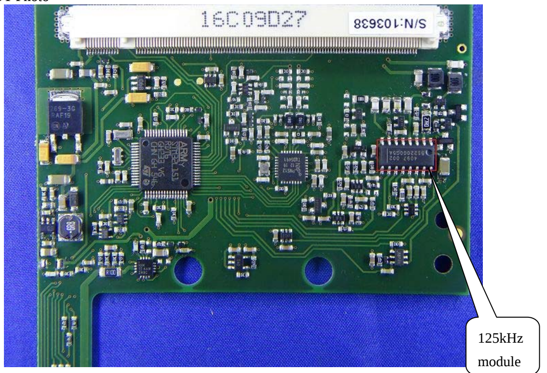
(18) EUT Photo
