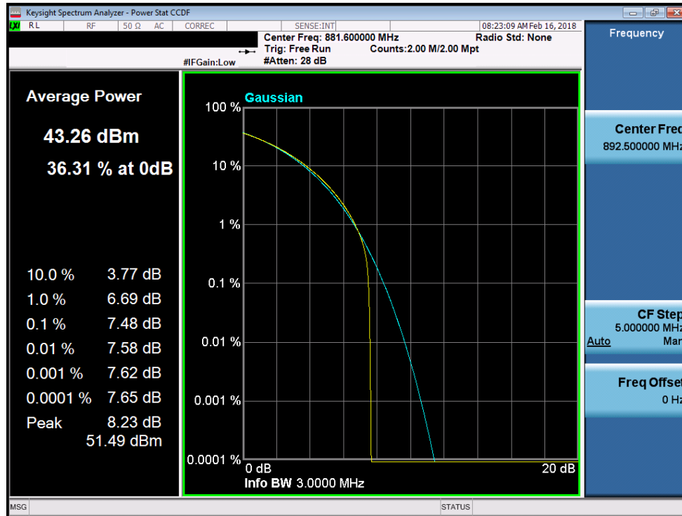
Plot 7-263. PAR Plot (Band 5 - 3.0MHz QPSK)
