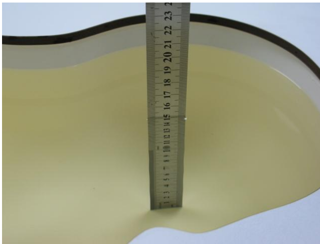
Photo 17: HSL 2450MHz depth (15cm)
