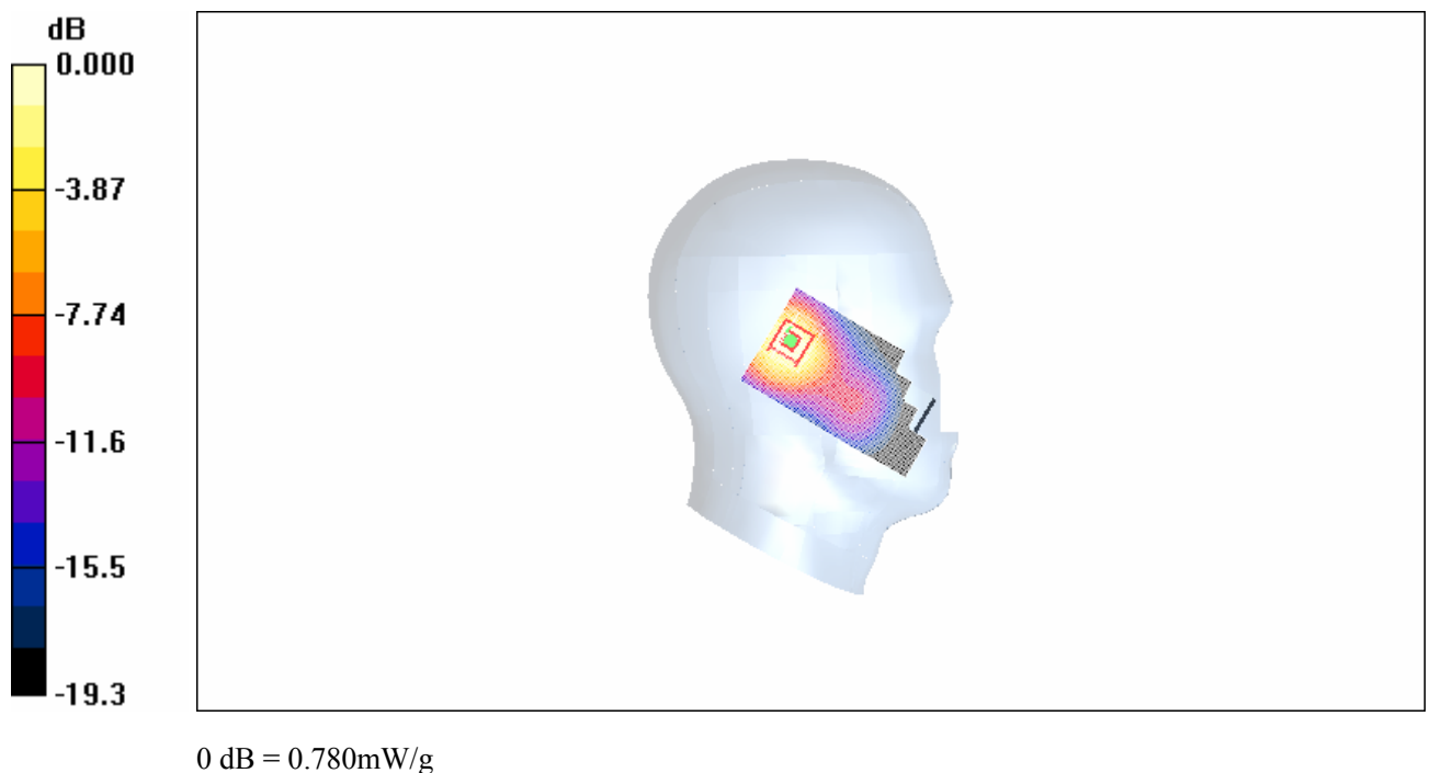
Fig. 9 Left Hand Tilt 15°PCS 1900MHz CH661
