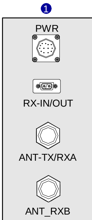
Module bottom
