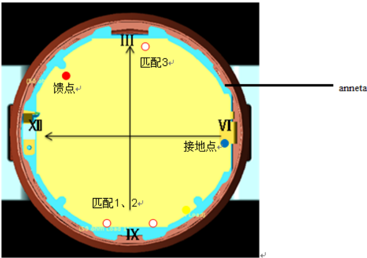
图（b）天线馈电点示意图
