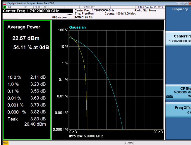
QPSK-20375
