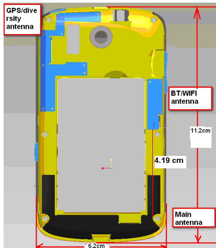
a: EUT
