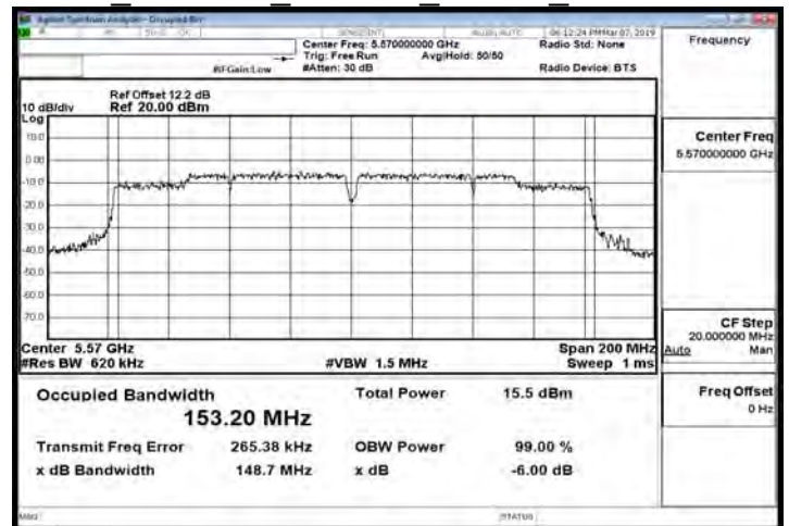
IC 802.11ac 160MHz Chain1 5570MHz
