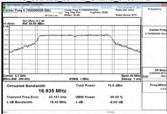
IC 802.11a 20MHz Chain1 5700MHz
