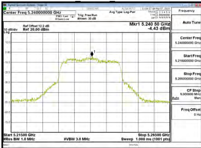
802.11n 20MHz 5240MHz
